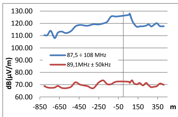
Фиг. 4. Измерени стойности за интензитета на електрическото поле в близост до точка TxP1
