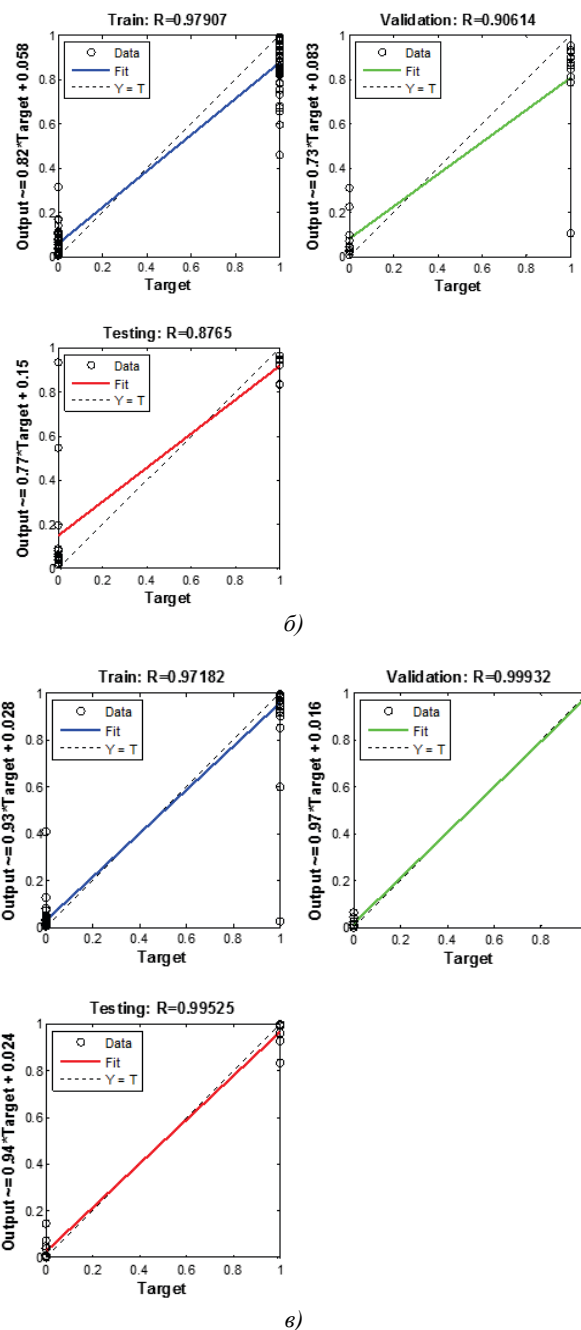
Фиг. 2. Линии на регресия за селектираните FFNNs за идентификация на географски зони на Интернет потребление при съотношения между невроните в скритите слоеве а) „1:1“, б) „1:2“ и в) „2:1“
