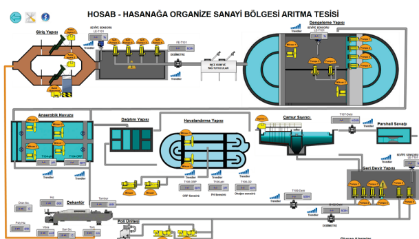
Fig. 1. HOSAB SCADA
