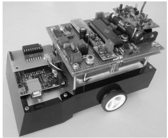
Фиг. 2. Прототип на мобилен безконтактен амперметър
